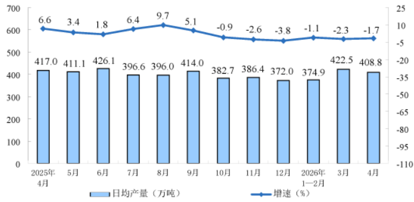
规模以上工业钢材同比增速及日均产量
